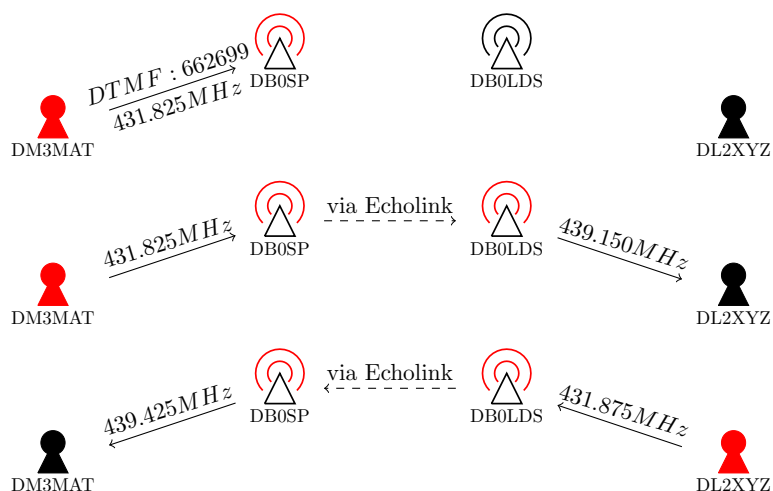
Abbildung 3: Repeaterbetrieb mit Echolink. DM3MAT verbindet die Repeater DB0SP (bei Berlin) und DB0LEI (bei Leipzig) per Echolink. Daraufhin können DM3MAT und DL2XYZ wie über einen gemeinsamen Repeater kommunizieren.
