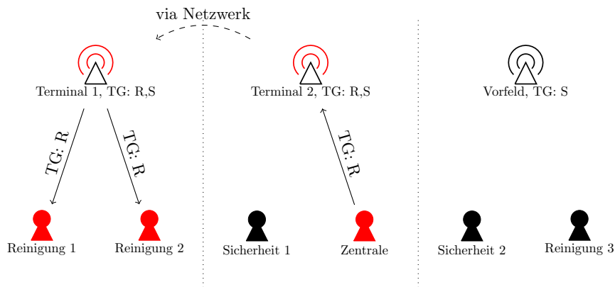
(a) Ein Gruppenruf zur Sprechgruppe Reinigung von der Zentrale aus. Der Teilnehmer Reinigung 3 wird aber nicht erreicht, da der Vorfeldrepeater diese Sprechgruppe nicht abonniert hat.
