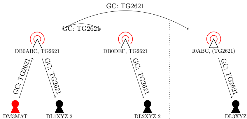
(b) Der OM im Ausland abonniert diese Sprechgruppe an dem lokalen Repeater temporär durch einen Gruppenruf zu dieser Sprechgruppe.
